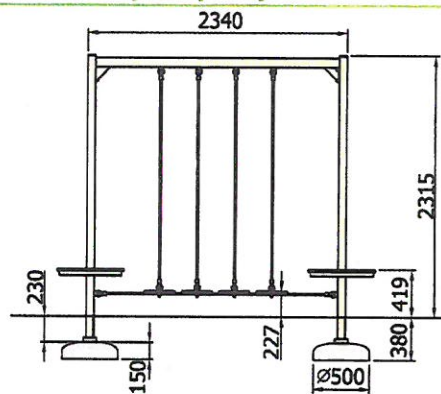
Wymiary urządzenia
